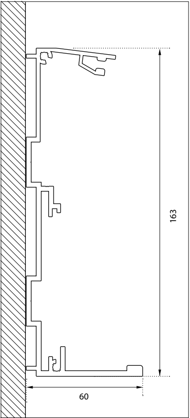
Wandprofil TR15 (Wandbefestigung)
