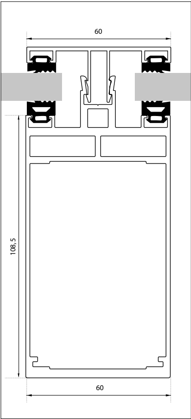
Querträger TR15
