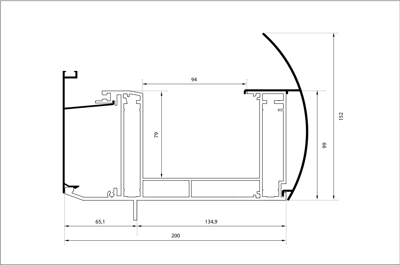
Rinne TR15 mit Rinnenblende RUND und Klickblende
