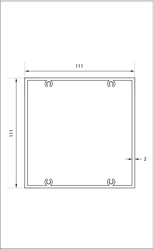
Querschnitt Pfosten TR15
